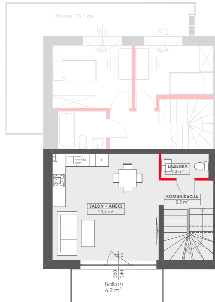
PIĘTRO
